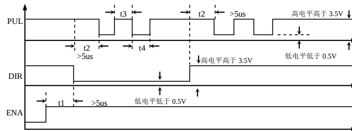
图 4 控制信号时序图
