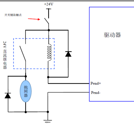
图 7 (a) 普通继电器接抱闸电机
