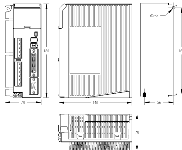
图 1 机械安装尺寸图(单位:mm)
