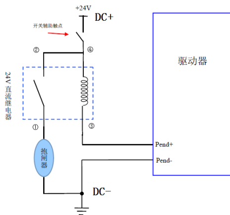
图 7 (b) 固态继电器接抱闸电机
