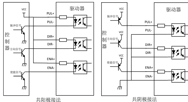
图 3(b) 单端方式控制信号接口接线图
