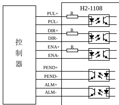
图 3(a) 差分方式控制信号接口接线图
