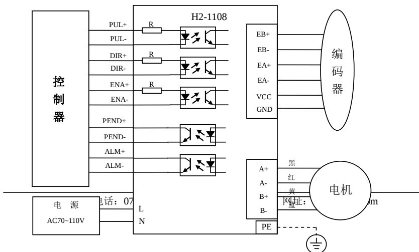
图 6 典型接线图
